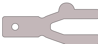
Part.# 8679 000 Distanzgabel „PVC“ für MOZART Abstoßmesser und SpeedTrimmer Spacer Claw „Vinyl“ for MOZART Trimmer and SpeedTrimmer
