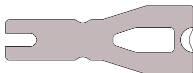
Part.# 8678 000 Ersatzklinge für MOZART Abstoßmesser und SpeedTrimmer Spare Blades for MOZART Trimmer and SpeedTrimmer
